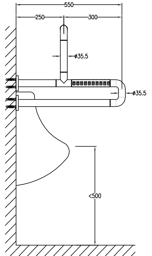
侧立面
