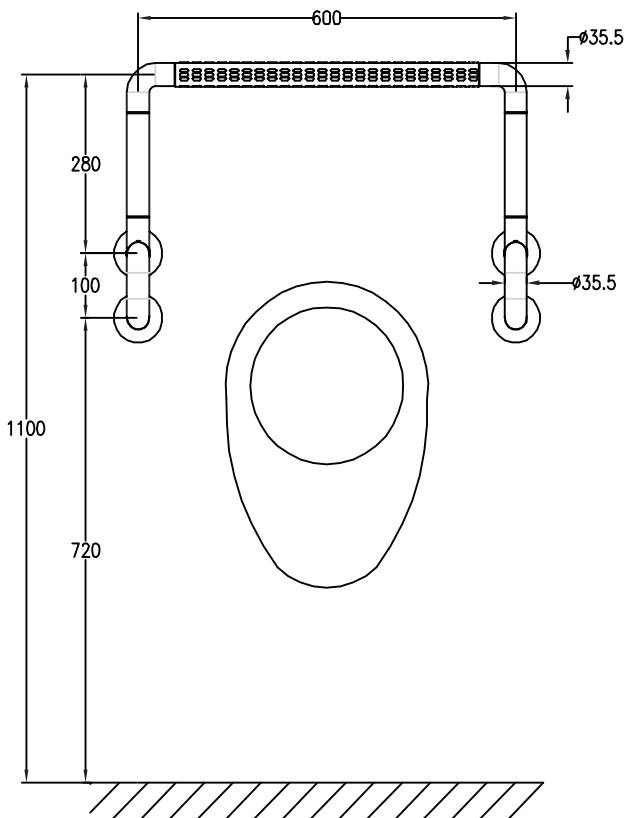
正立面
